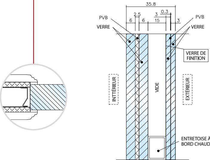
Avec double vitrage isolant de 35,8 mm anti-effraction
