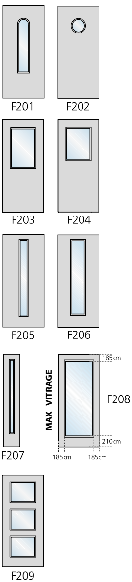
Avec double vitrage isolant de 35,8 mm anti-effraction
