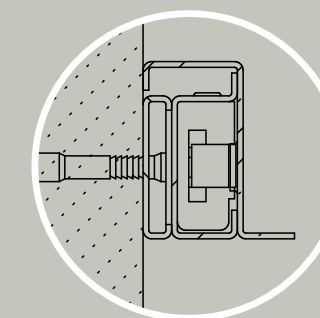
SISTEMA DI FISSAGGIO DEL TELAIO ACCOPIATO AL CONTROTELAIO TRAMITE TASSELLO CHIMICO
