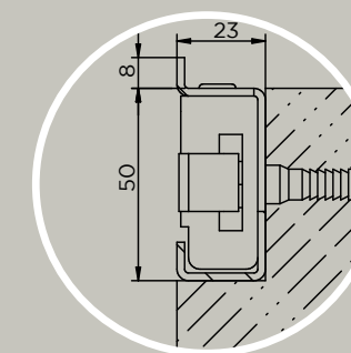
SISTEMA DI FISSAGGIO TRADIZIONALE CON LA MURATURA DEL CONTROTELAIO
